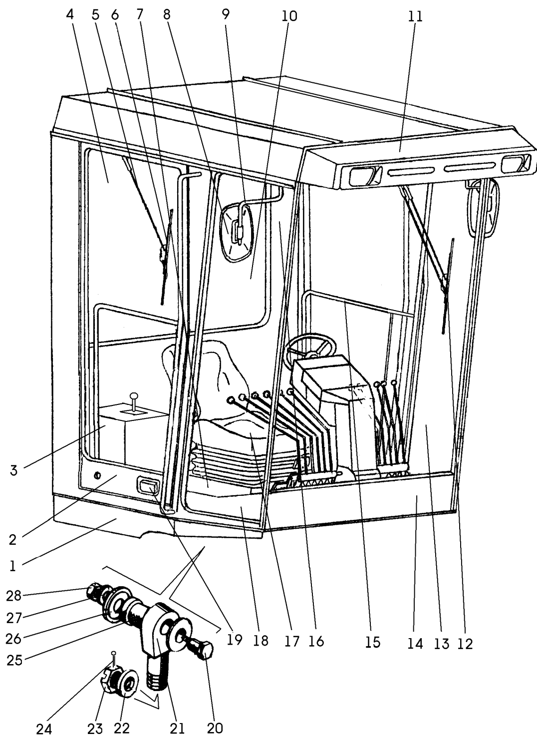
Рисунок 2.10.1 – Кабина А122Б-1.33.00.000-03
