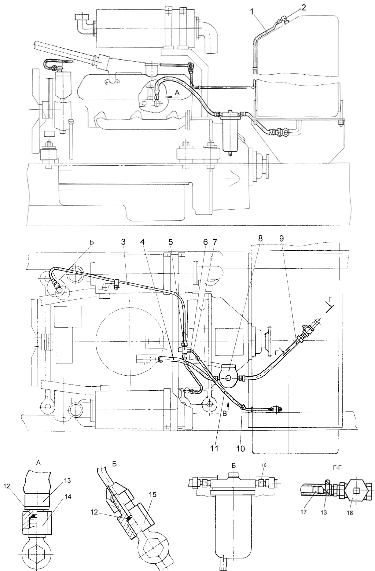
Рисунок 2.1.7 - Топливопроводы ДЗ-122Б-6.10.06.000
