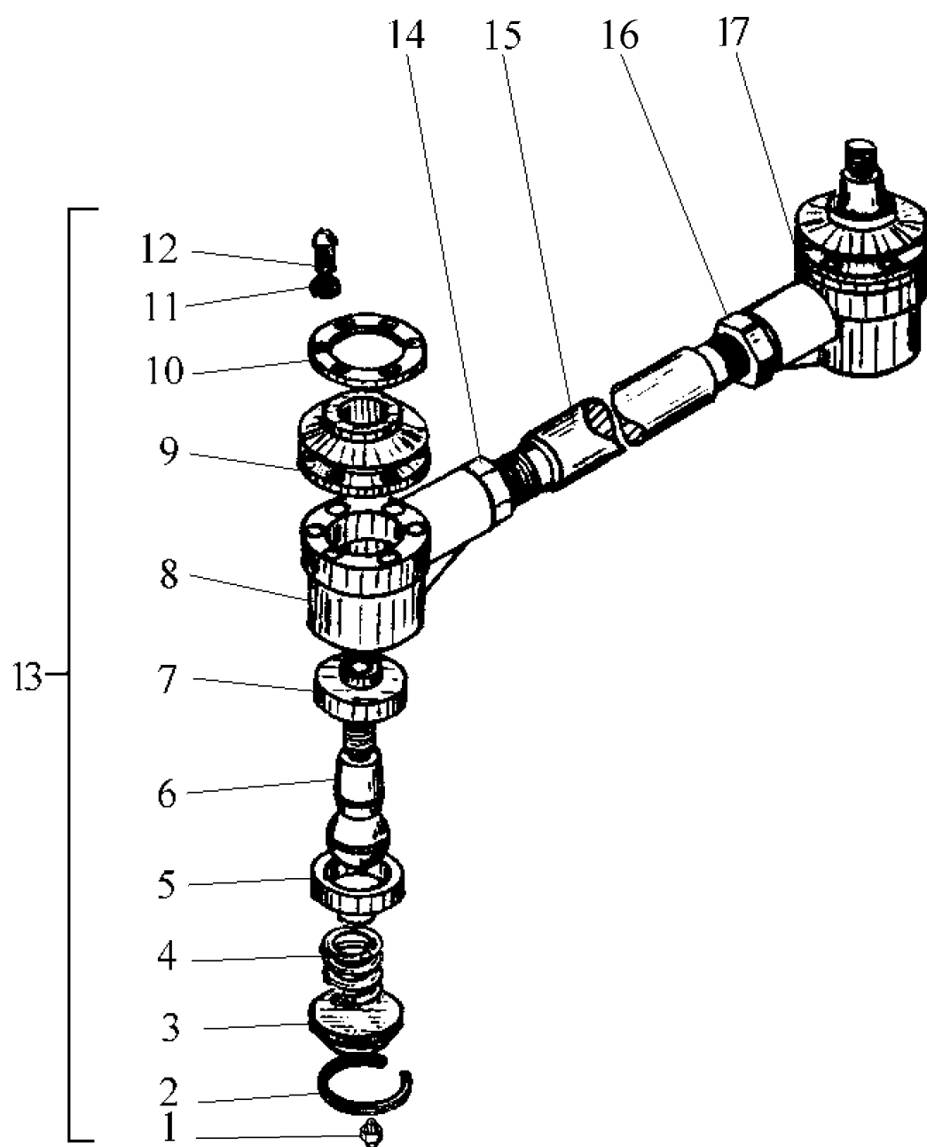
Рисунок 2.6.2 – Тяга ДЗ-122Б.03.09.000
