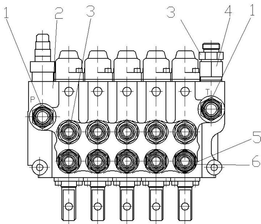
Рисунок 2.8.15 - Гидрораспределитель ДЗ-122Б-7.79.01.010-01
