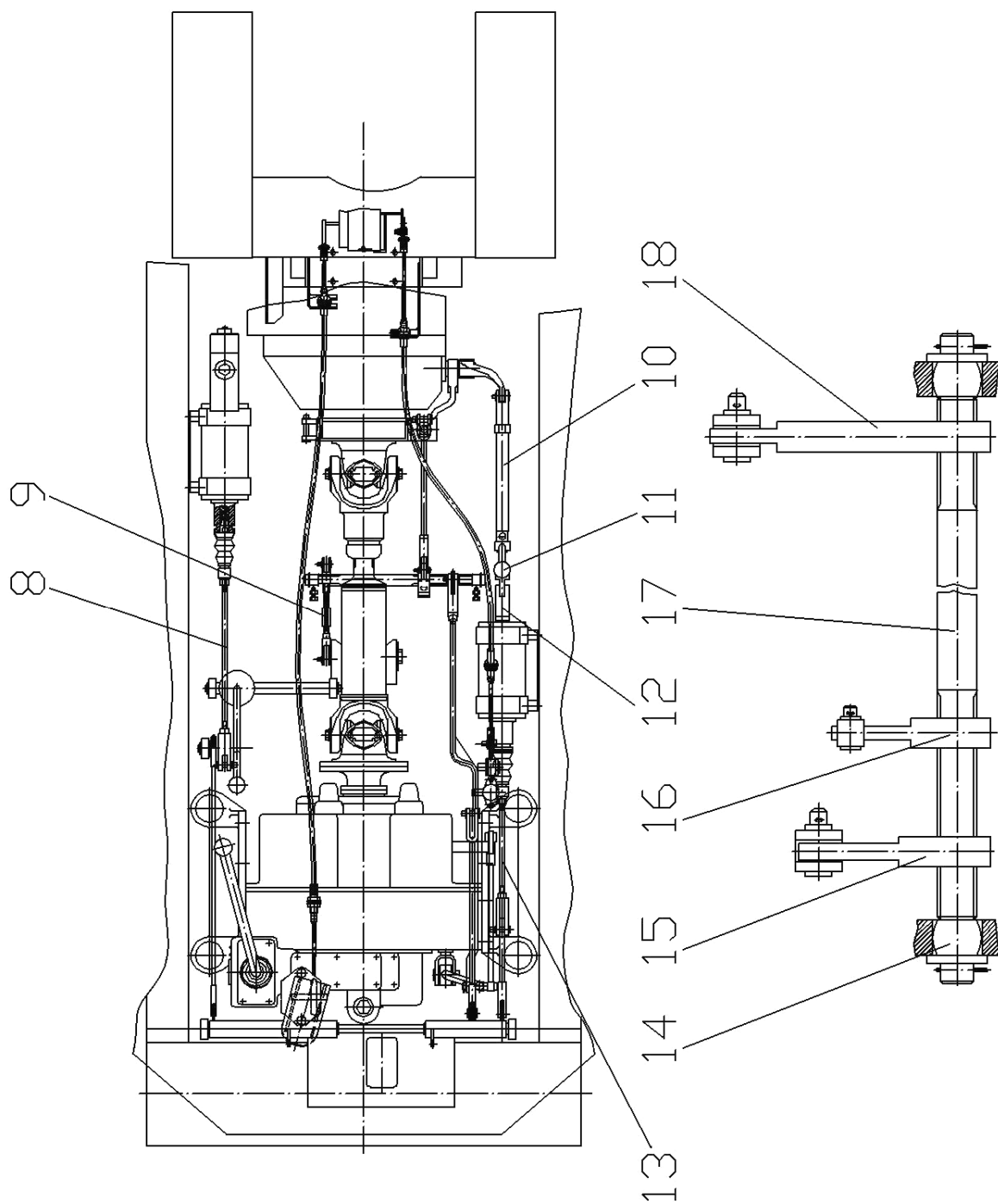
Рисунок 2.10.6 – Привод А122Б-7.33.43.000 (продолжение)
