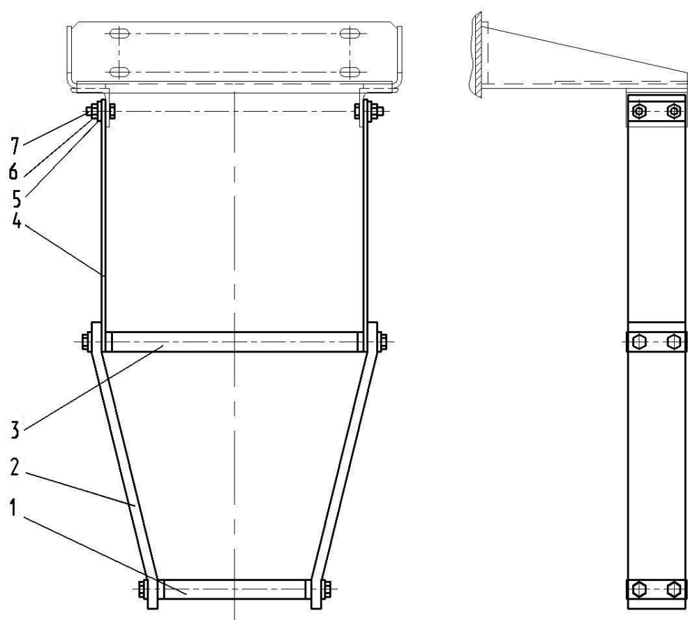
Рисунок 2.4.5 Лестница ДЗ-122Б.53.00.000
