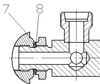
Рисунок 2.8.16 - Гидрораспределитель ДЗ-122Б-7.79.01.020
