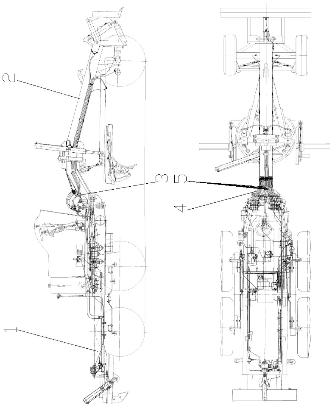
Рисунок 2.8.5 - Гидропривод ДЗ-122Б-7.79.00.000-03
