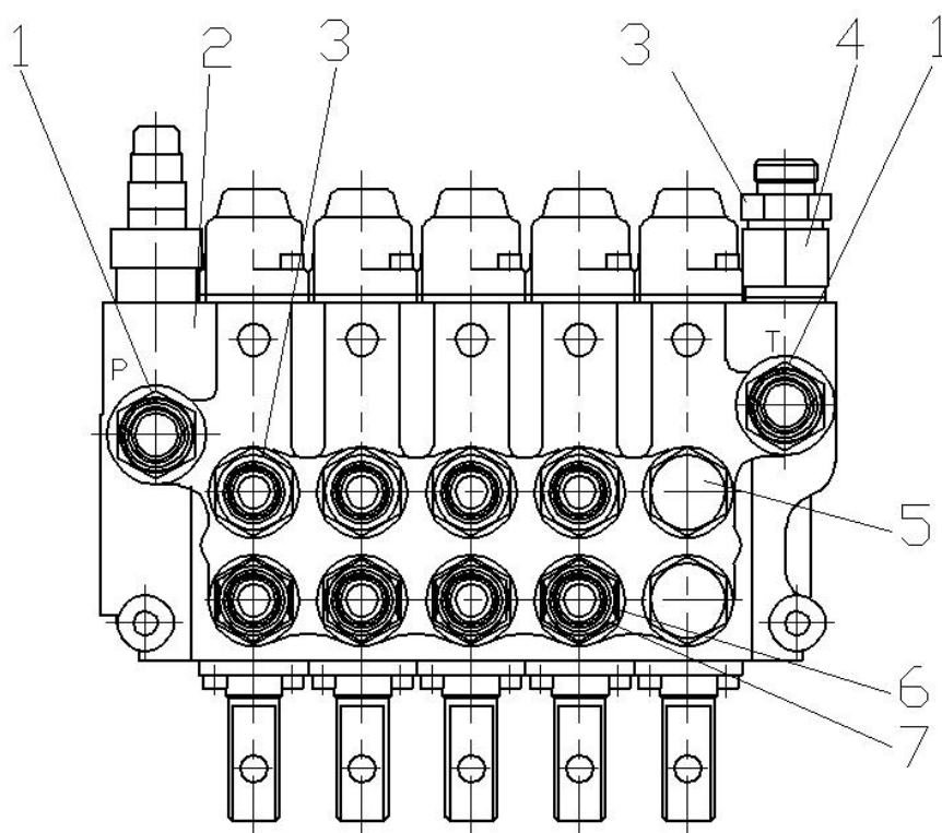
Рисунок 2.8.14 - Гидрораспределитель ДЗ-122Б-7.79.01.010
