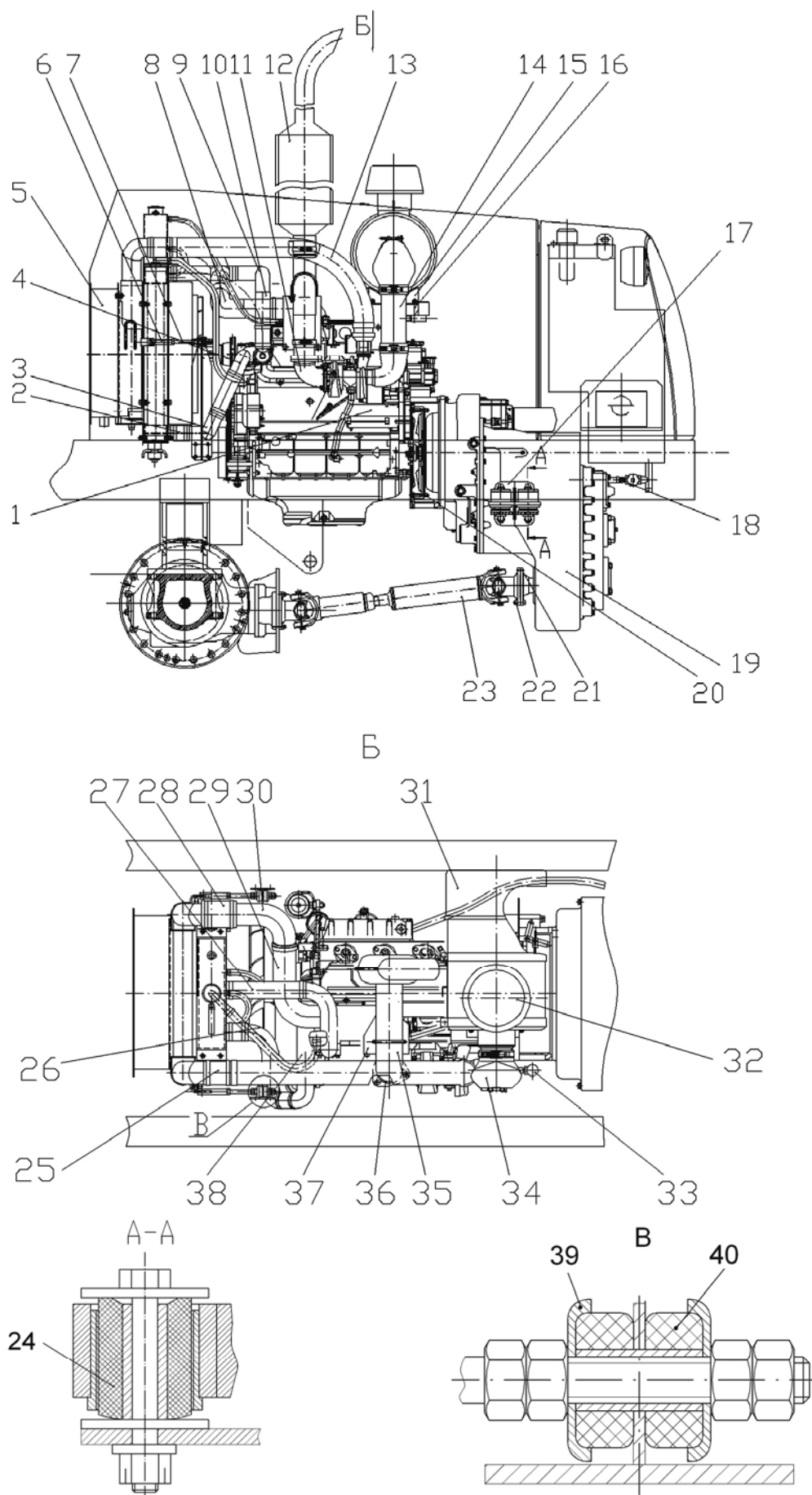
Рисунок 2.1.1 – Агрегат силовой А122Б-2.10.00.000
